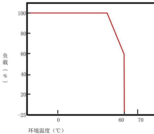
温度特性(降额)曲线
