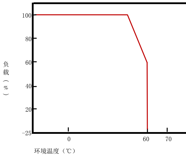
温度特性(降额)曲线
