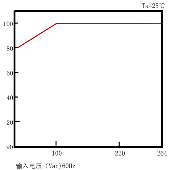
静态特性曲线
