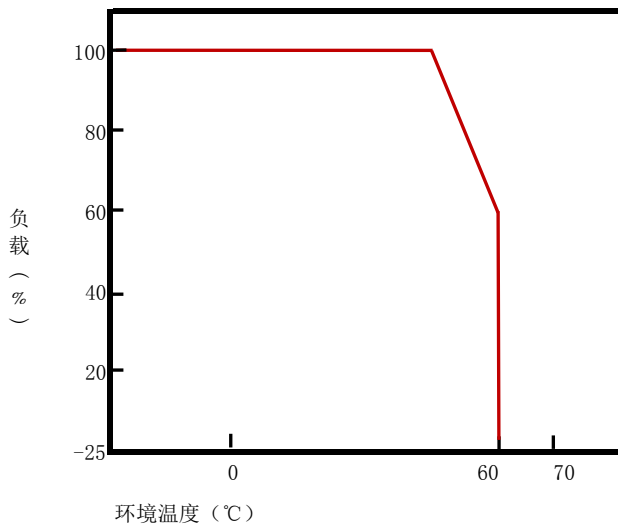
温度特性(降额) 曲线
