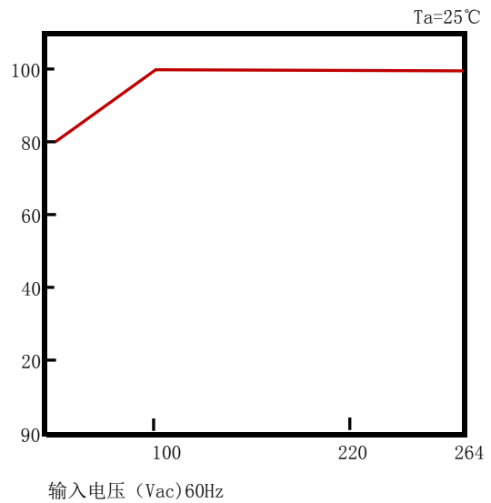
静态特性曲线
