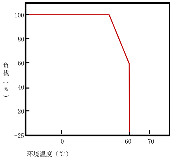
温度特性(降额) 曲线
